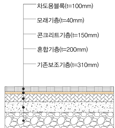
콘크리트기층 포장
